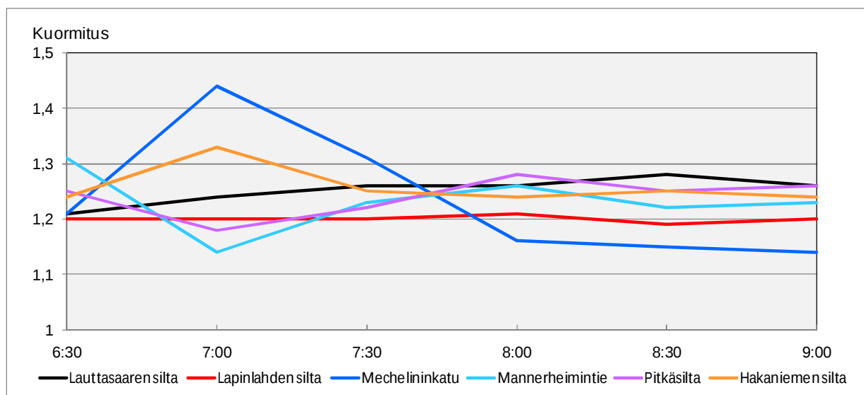
Kuva 3. Keskiakuormituksen vaihtelu puolitunneittain laskentapisteissä aamuliikenteessä keskustan suuntaan klo 6-9
