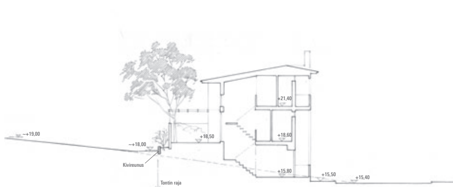
Kortteli 31206, leikkaus 1/300
