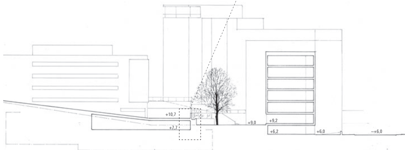
Alueen periaateleikkaus
