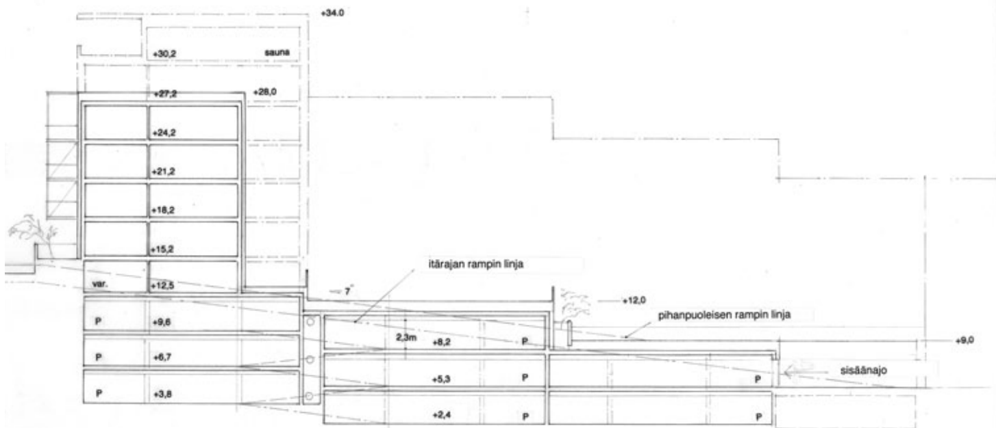
Pysäköintilaitos, periaateleikkaus
