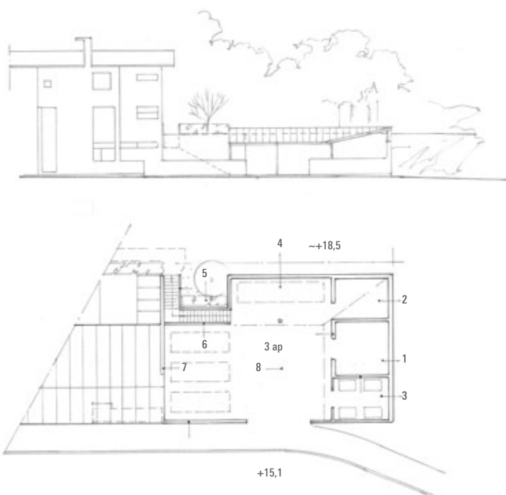
Kortteli 31206, huoltorakennus 1/200
