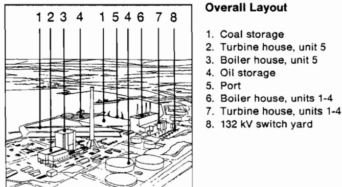
Kuva 1. Asnäsin kivihiilivoimalaitos.
