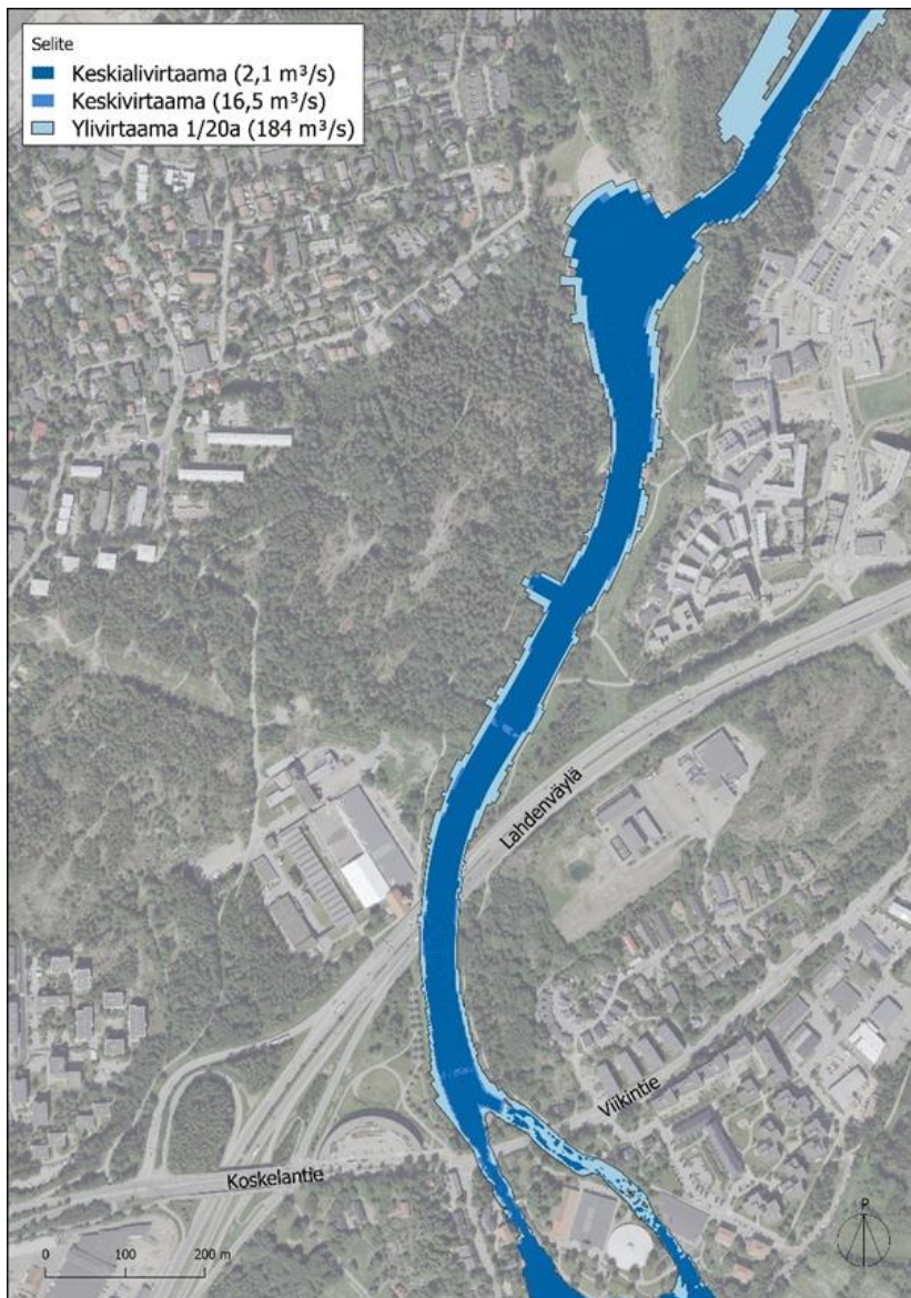
Kuva 31 Simuloidut vedenkorkeudet skenaariossa 4 Vanhankaupunginkosken Pikkukosken uimarannan välillä (keskiäli-, keski- ja ylivirtaama).
