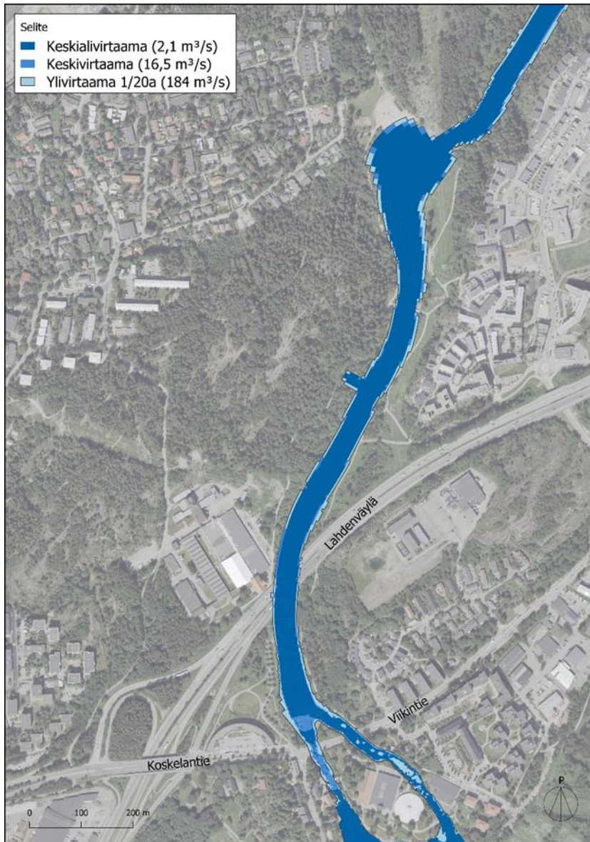
Kuva 29 Simuloidut vedenkorkeudet skenaariossa 3 Vanhankaupunginkosken Pikkukosken uimarannan välillä (keskiali-, keski- ja ylivirtaama).
