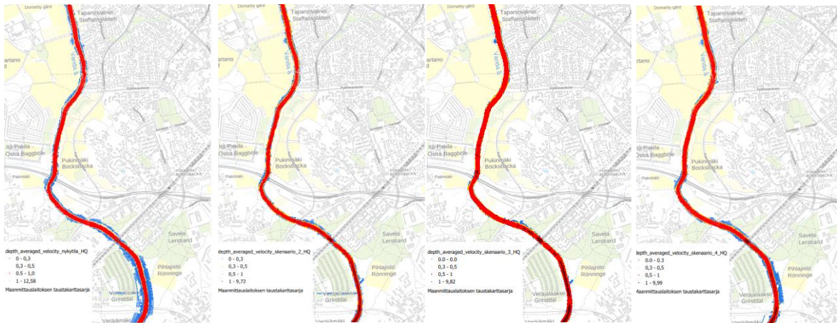
Kuva 37 Keskiosan virtausnopeudet HQ-tilanteessa. Skenaariot vasemmalta oikealle: 1,2,3 ja 4. Siniset pisteet: kerrostumialue. Keltaiset pisteet: akkumulaatioalue. Punaiset pisteet: eroosioalue. Viininpunaiset pisteet: eroosioalue, virtausnopeus yli 1 m/s.
