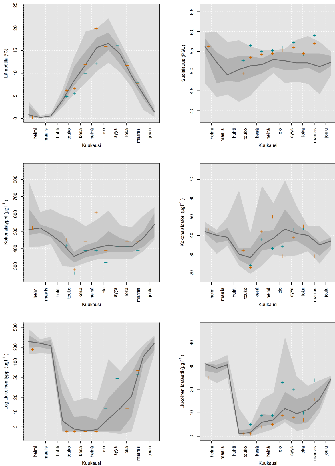
Kuva 13. Villinki -vesimuodostuman pohjanläheisen veden (pohja +1 m) havaintojen kuukausikoh- taiset viimeisen 20 vuoden mediaanit sekä 5., 25., 75. ja 95. persentiilit ja kulu- van vuoden havainnot. Kuva jatkuu seuraavalla sivulla.
