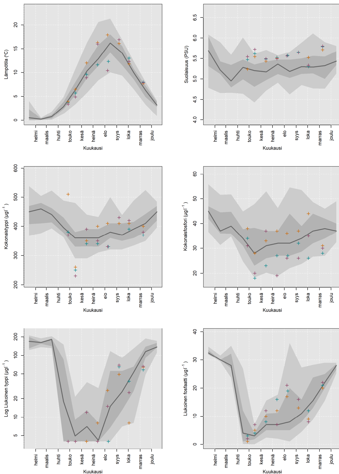
Kuva 15. Sipoon saaristo vesimuodostuman pohjanläheisen veden (pohja +1 m) havaintojen kuukausikohtaiset viimeisen 20 vuoden mediaanit sekä 5., 25., 75. ja 95. persentiilit ja kuluvan vuoden havainnot. Kuva jatkuu seuraavalla sivulla.
