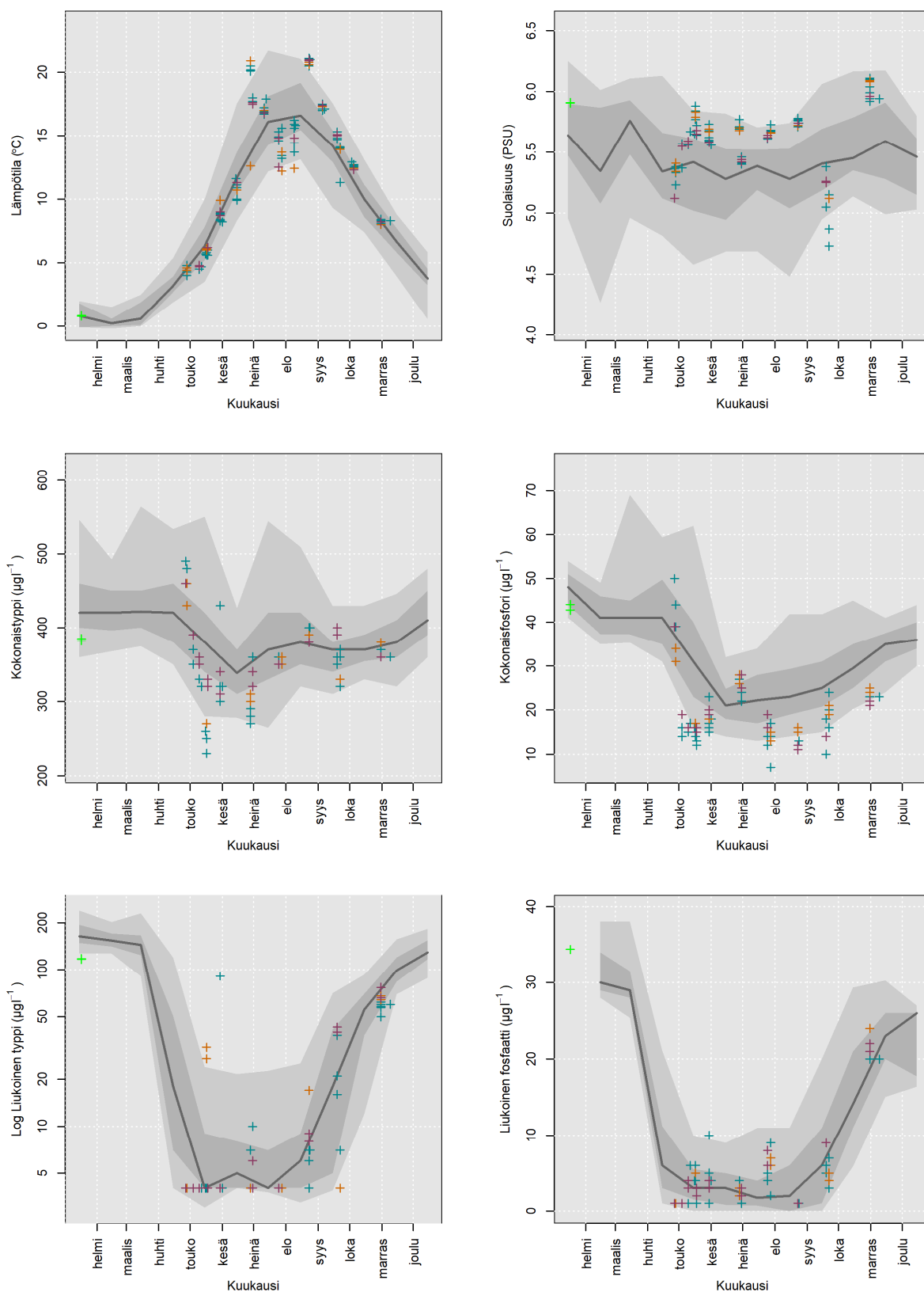
Kuva 2. Helsinki-Porkkala vesimuodostuman pintaveden havaintojen kuukausikohtaiset viimeisen 20 vuoden mediaanit sekä 5., 25., 75. ja 95. persenttiit ja kuluva vuoden havainnot. Kuva jatkuu seuraavalla sivulla.
