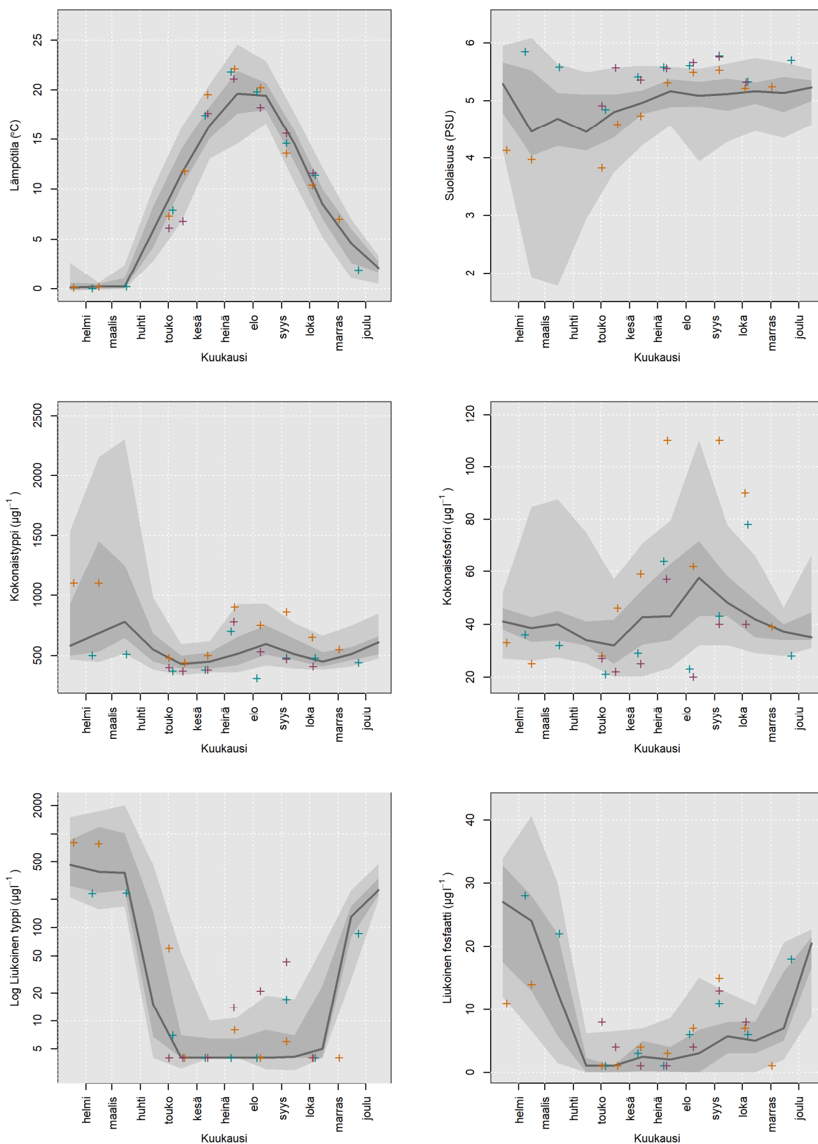
Kuva 8. Seurasaari vesimuodostuman pintaveden havaintojen kuukausikohtaiset viimeisen 20 vuoden mediaanit sekä 5., 25., 75. ja 95. persenttiit ja kuluva vuoden havainnot. Kuva jatkuu seuraavalla sivulla.
