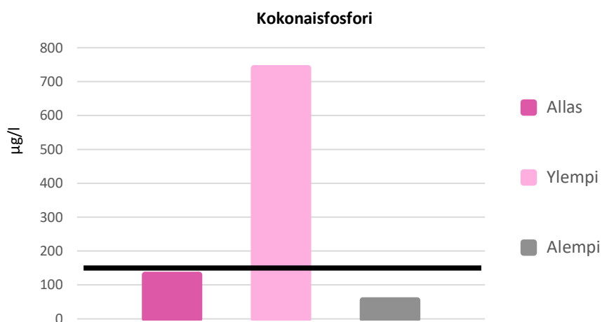
Kuva 3.3 Havaintopisteiden kokonaisfosforipitoisuus. Puhdistetun jäteveden pitoisuus 150 µg/l.
