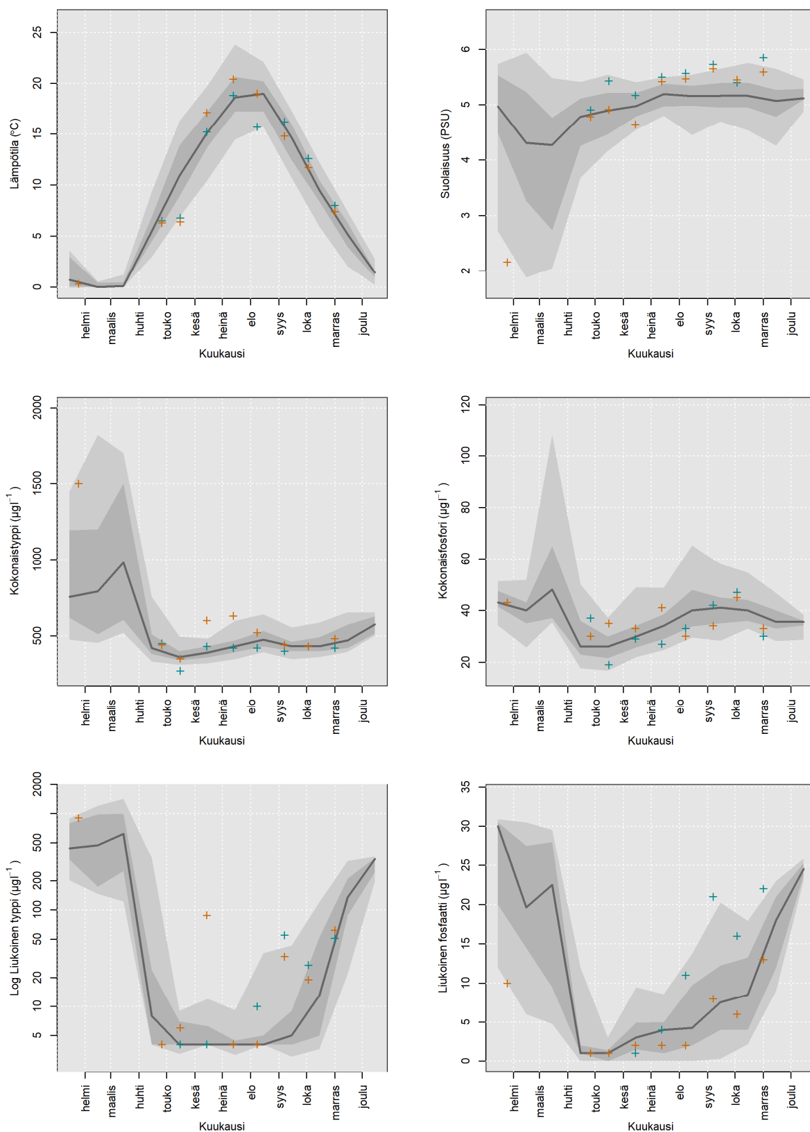
Kuva 12. Villinki -vesimuodostuman pintaveden havaintojen kuukausikohtaiset viimeisen 20 vuoden mediaanit sekä 5., 25., 75. ja 95. persentiilit ja kuluva vuoden havainnot. Kuva jatkuu seuraavalla sivulla.
