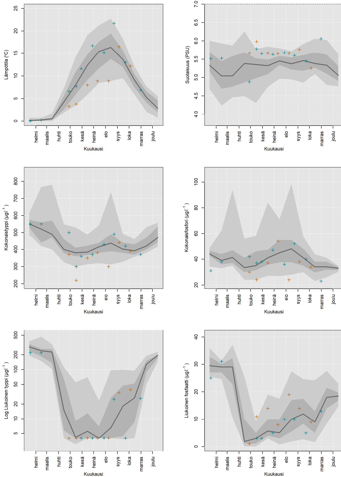
Kuva 7. Suvisaaristo-Lauttasaari vesimuodostuman pohjanläheisen veden (pohja +1 m) havaintojen kuukausikohtaiset viimeisen 20 vuoden mediaanit sekä 5., 25., 75. ja 95. persenttiit ja kuluva vuoden havainnot. Kuva jatkuu seuraavalla sivulla.
