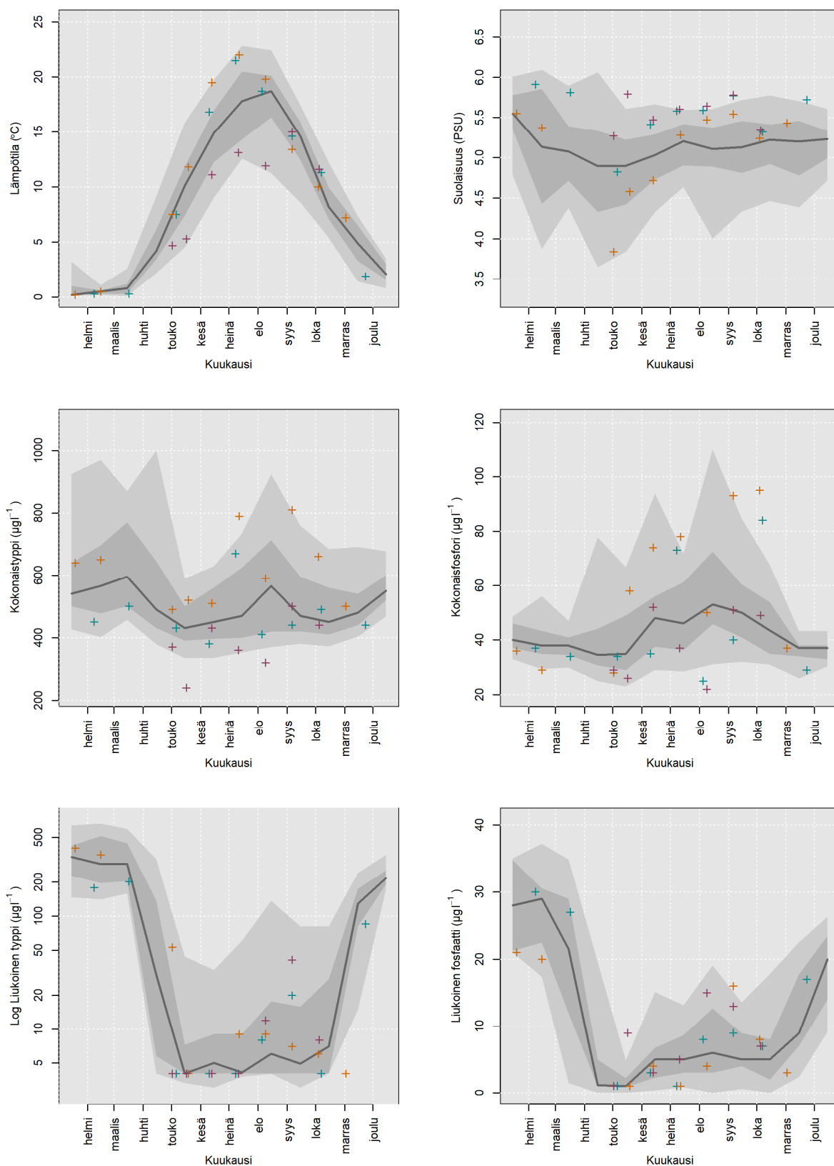
Kuva 9. Seurasaari vesimuodostuman pohjanläheisen veden (pohja +1 m) havaintojen kuukausi-kohtaiset viimeisen 20 vuoden mediaanit sekä 5., 25., 75. ja 95. persenttiit ja kuluva vuoden havainnot. Kuva jatkuu seuraavalla sivulla.
