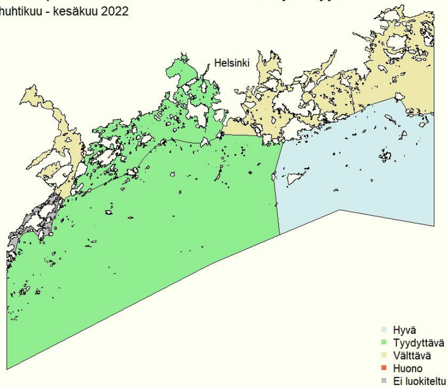
Kuva 16. Pääkaupunkiseudun merialueen vesimuodostumien rehevöityneisyyden tila vuoden 2022 vuosineljänneksillä. Luokittelu perustuu TRIX-trofiaiindeksiin. Kuva jatkuu seuraavalla sivulla.
