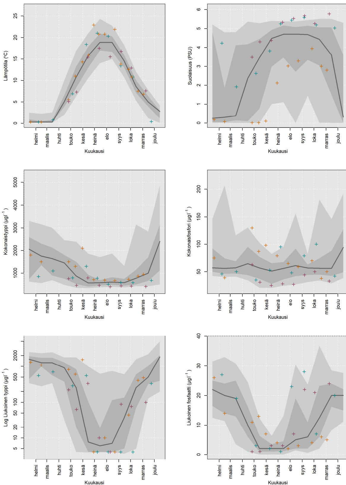
Kuva 10. Kruunuvuorenselkä vesimuodostuman pintaveden havaintojen kuukausikohtaiset viimeisen 20 vuoden mediaanit sekä 5., 25., 75. ja 95. persenttiit ja kuluva vuoden havainnot. Kuva jatkuu seuraavalla sivulla.
