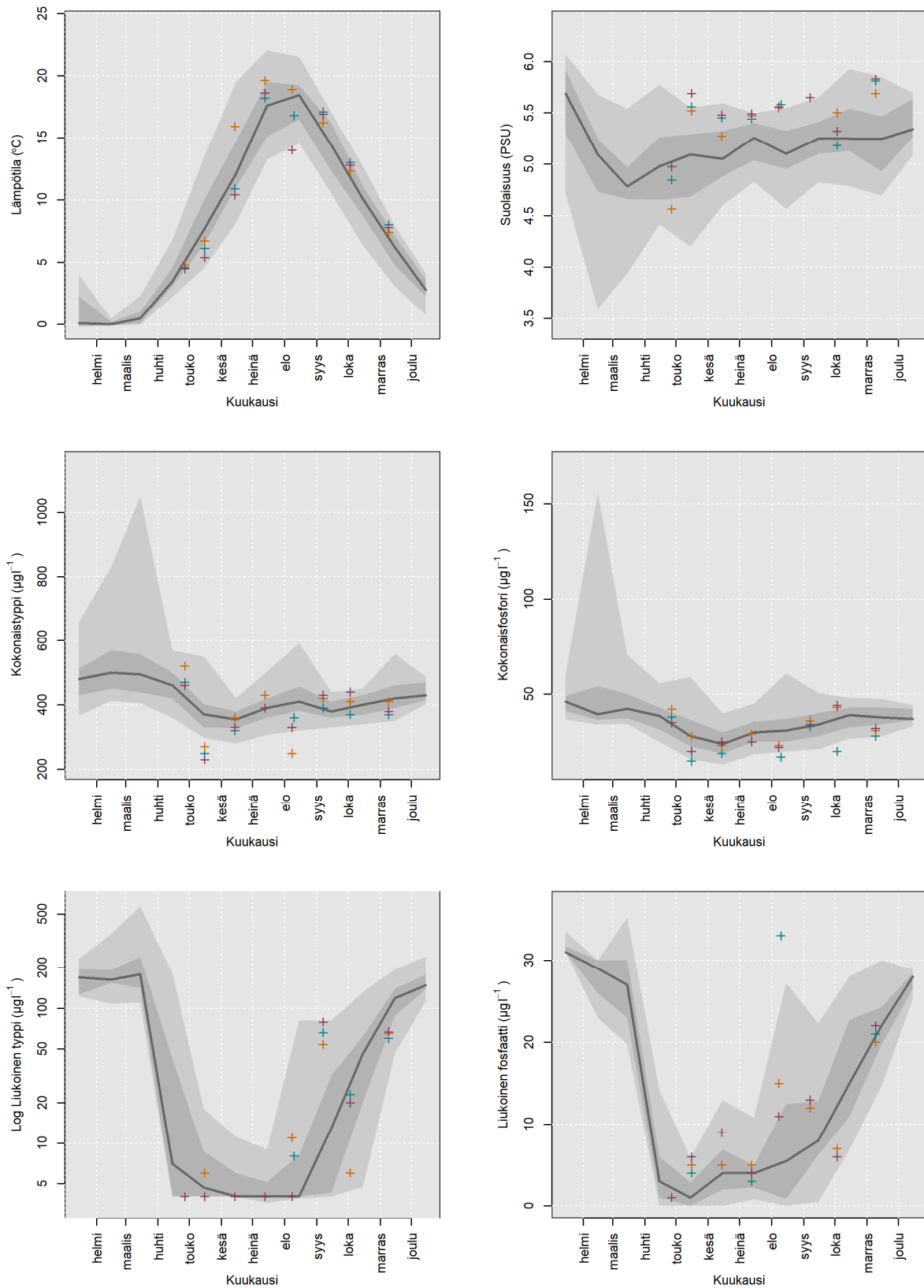
Kuva 14. Sipoon saaristo vesimuodostuman pintaveden havaintojen kuukausikohtaiset viimeisen 20 vuoden mediaanit sekä 5., 25., 75. ja 95. persenttiit ja kuluva vuoden havainnot. Kuva jatkuu seuraavalla sivulla.
