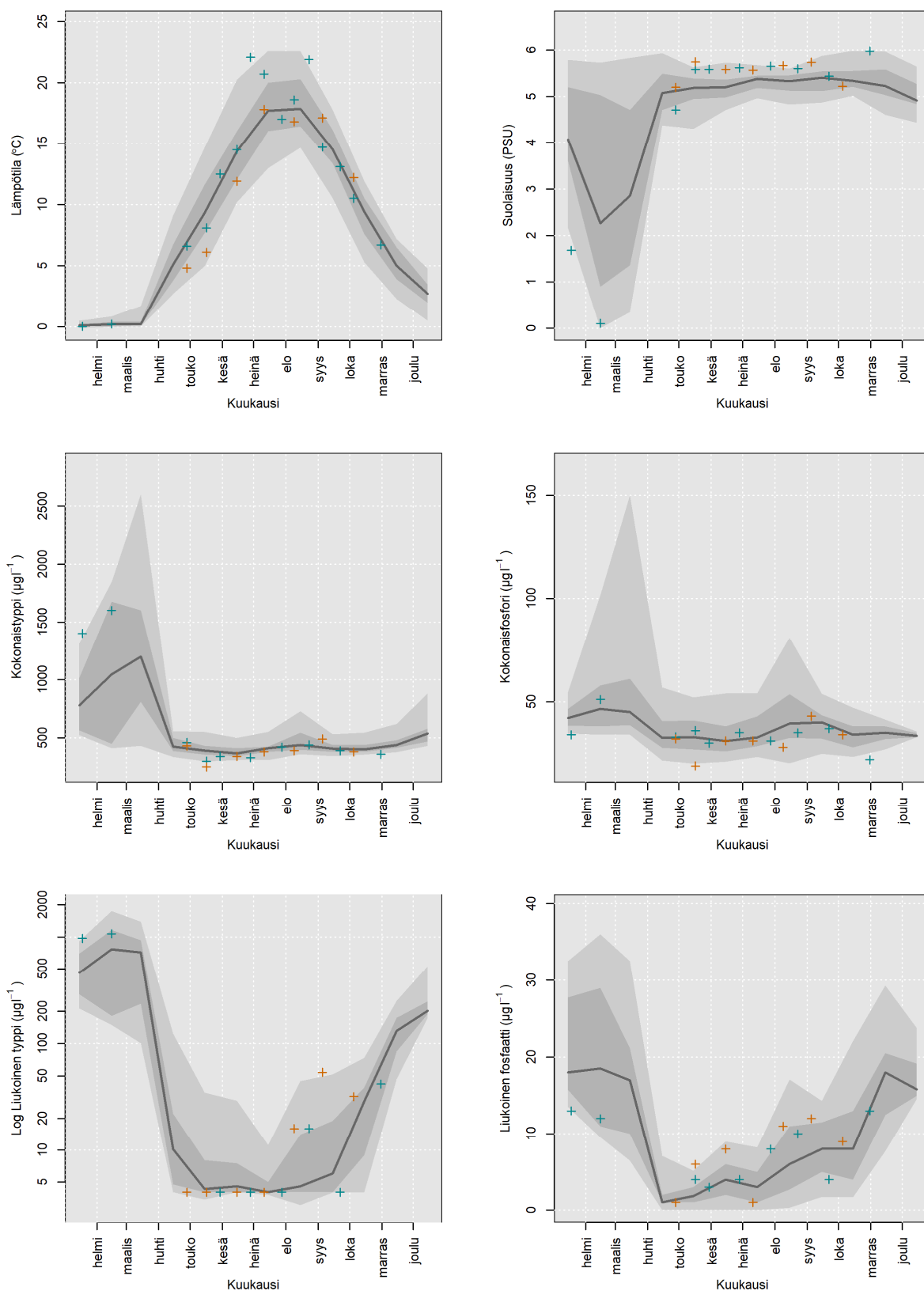
Kuva 6. Suvisaaristo-Lauttasaari vesimuodostuman pintaveden havaintojen kuukausikohtaiset vii-meisen 20 vuoden mediaanit sekä 5., 25., 75. ja 95. persentiilit ja kuluvan vuoden havainnot. Kuva jatkuu seuraavalla sivulla.
